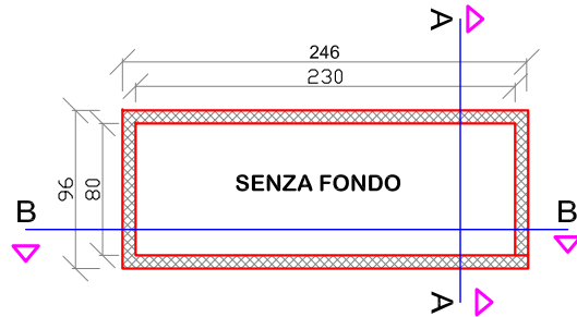
PIANTA LOCULO
