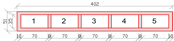
SEZIONE A-A
