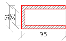
SEZIONE B-B
