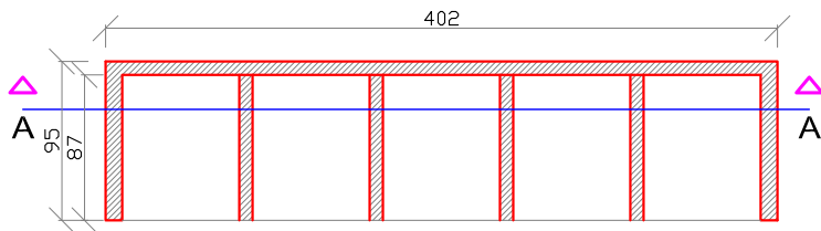
PIANTA
