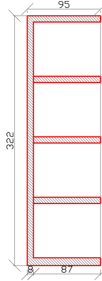
SEZIONE B-B
