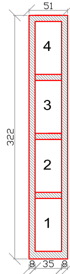
SEZIONE A-A
