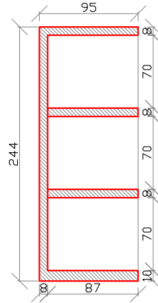
SEZIONE B-B
