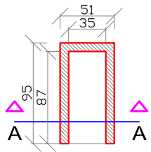
PIANTA
