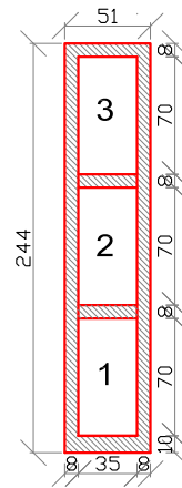
SEZIONE A-A
