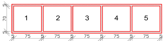
SEZIONE A-A
