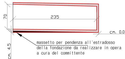
SEZIONE B-B
