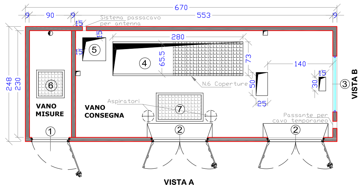
PIANTA CABINA DI CONSEGNA
