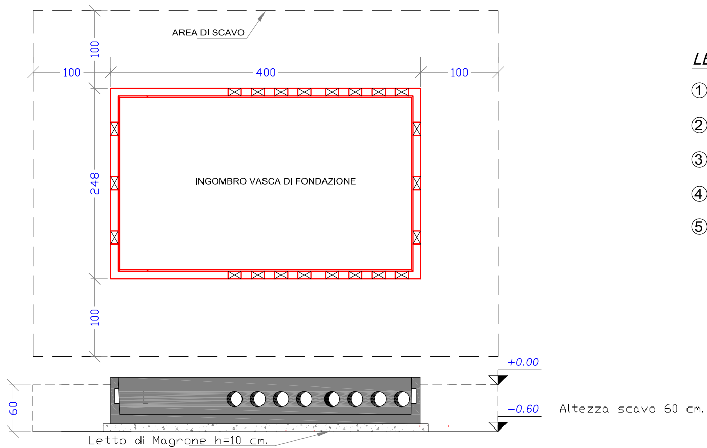
DIMENSIONI SCAVO PER ALLOGGIAMENTO VASCA DI FONDAZIONE
