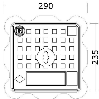
PIANTA CHIUSINO
