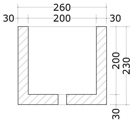
SEZIONE POZZETTO
