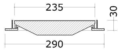
SEZIONE CHIUSINO
